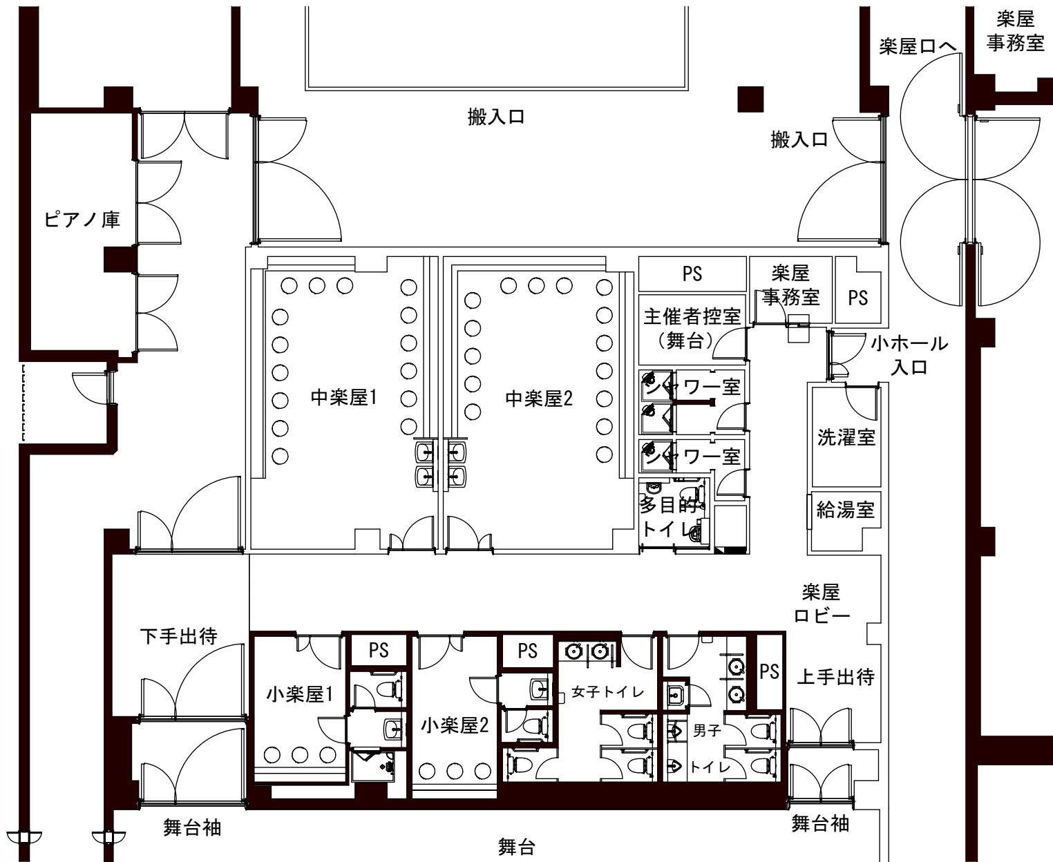
小ホール楽屋平面図
